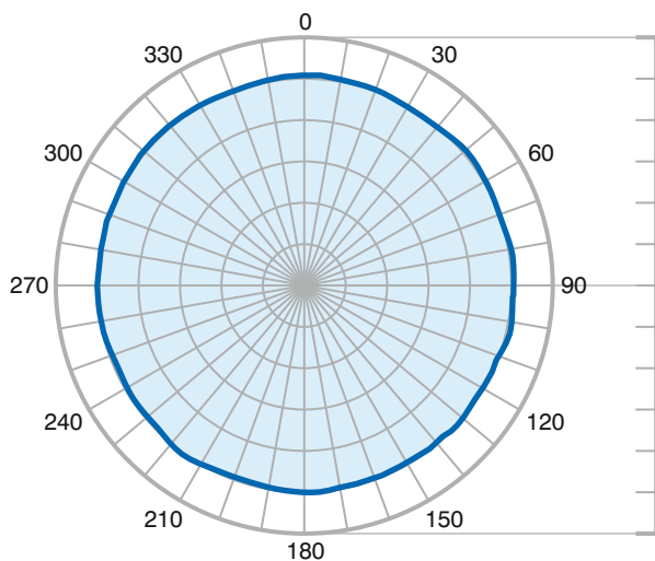
Horizontal @ 5.8GHz
